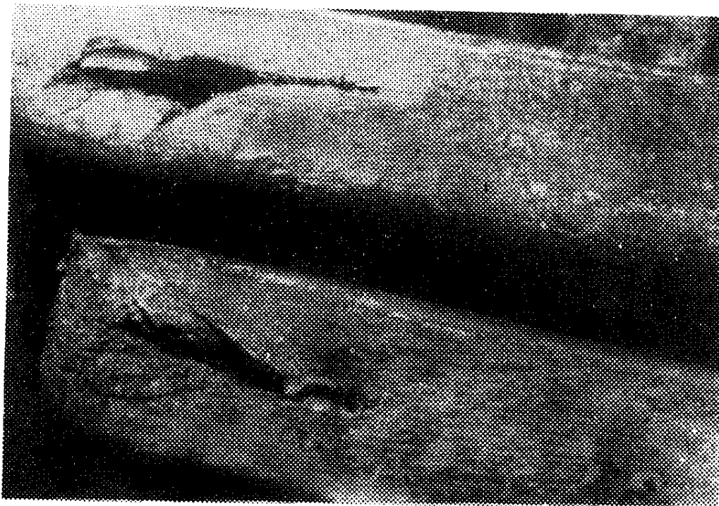
17. Скворечник (внешний вид)
